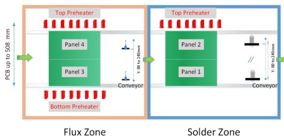
Integra™ 508.2PD-Konfiguration
