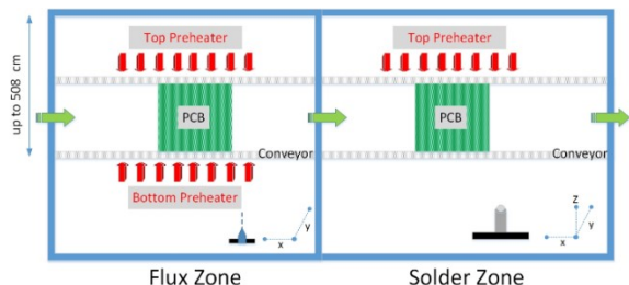
Integra™ 508.2S-Konfiguration
